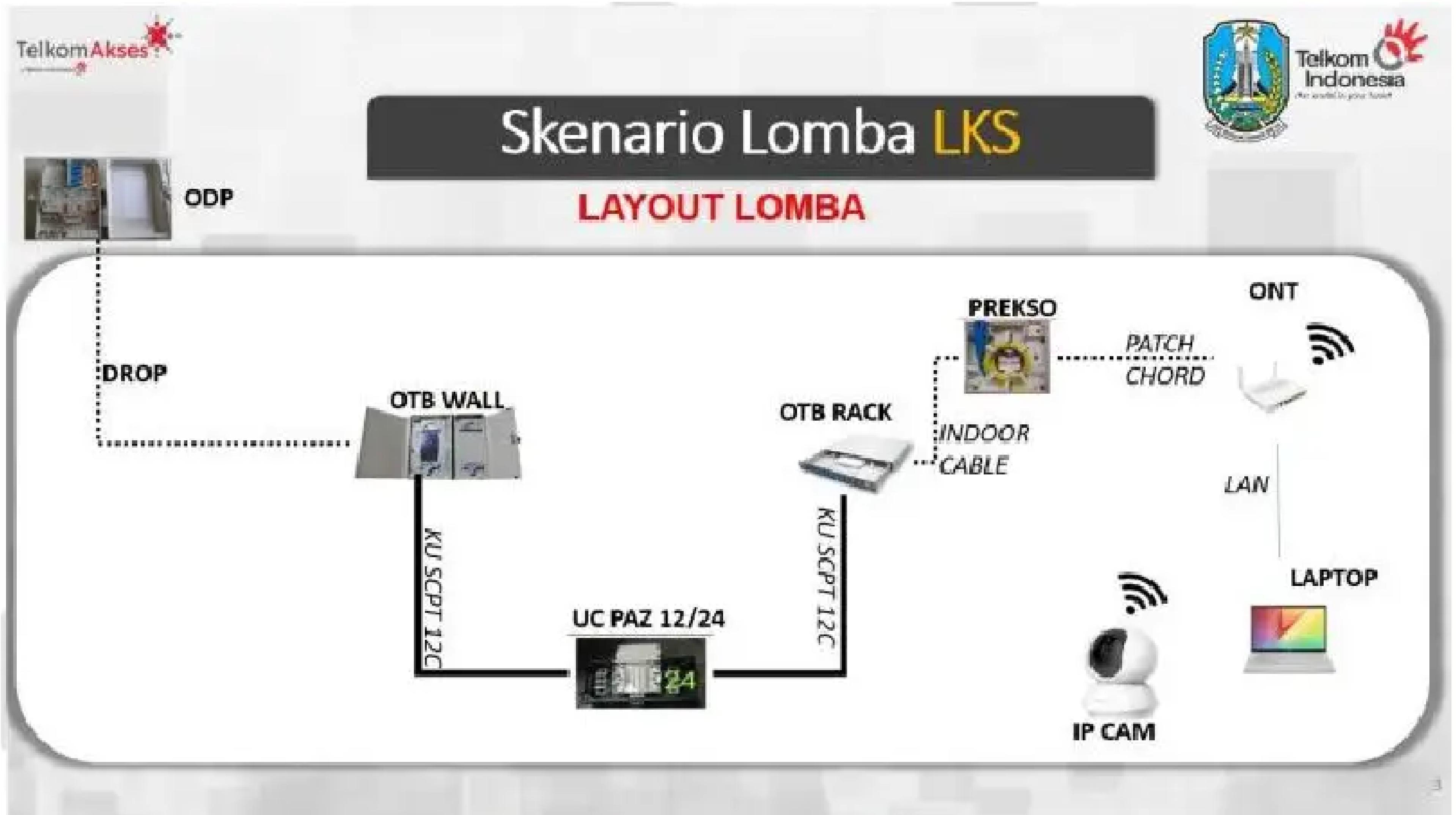
Gambar 1. Layout keseluruhan
